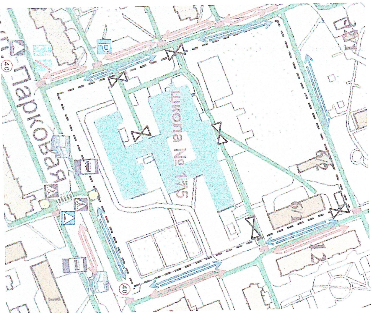
Схема организации дорожного движения в непосредственной близости от образовательной организации с размещением соответствующих технических средств организации дорожного движения, маршруты движения детей и расположение парковочных мест.
